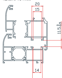
適合材断面
