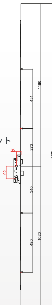
2200/92/35 mm キー操作式多点ロック（バックセット35 mm）
